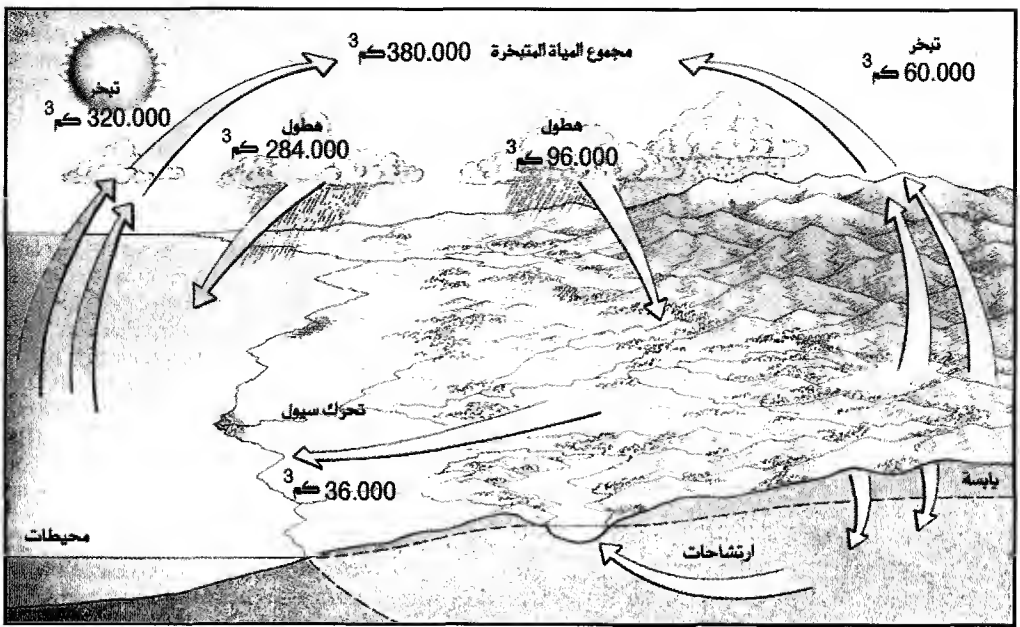
رسم تخطيطي يوضح دورة الماء حول الأرض
